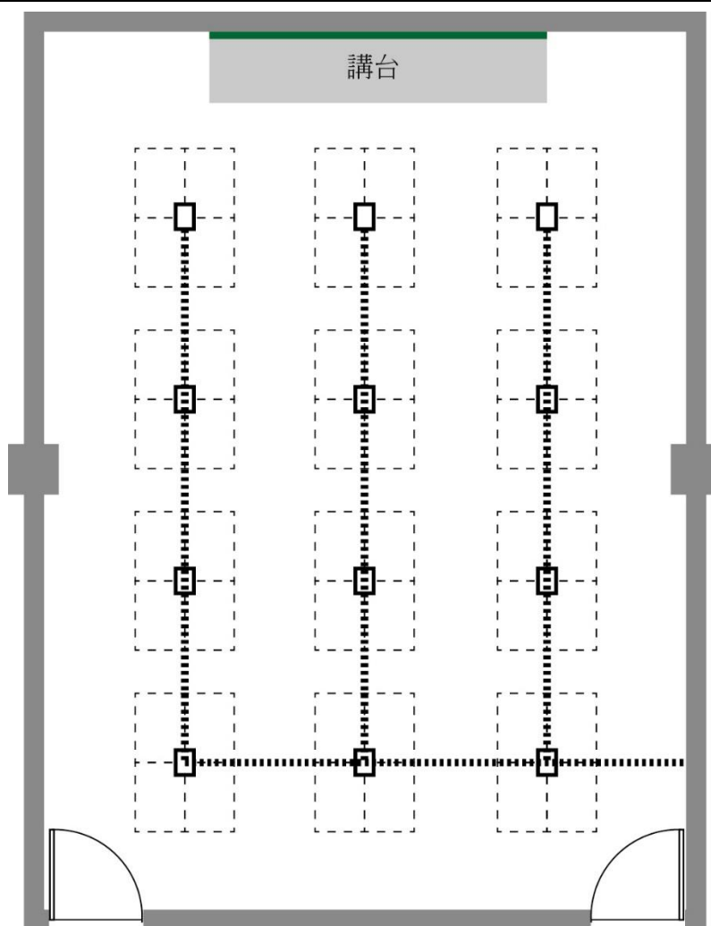
自強 409 設計教室改善示圖
